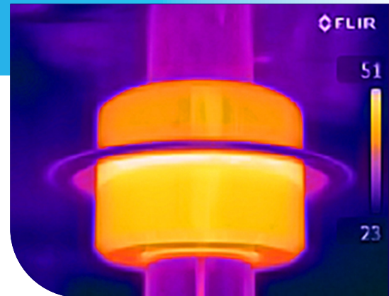
Die SeccoMix R, aufgenommen mit einer Wärmebildkamera. Die Temperaturwerte lagen deutlich unter den zugelassenen Werten der Temperaturklasse T4.
